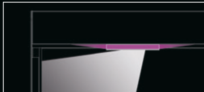
Secção vertical wallwasher LD7-LED-RGB Esquema funcional iluminação direta e indireta
