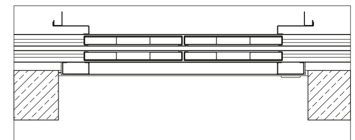
Secção horizontal das portas da cabina e da caixa com aros / Remate de parede T1.
