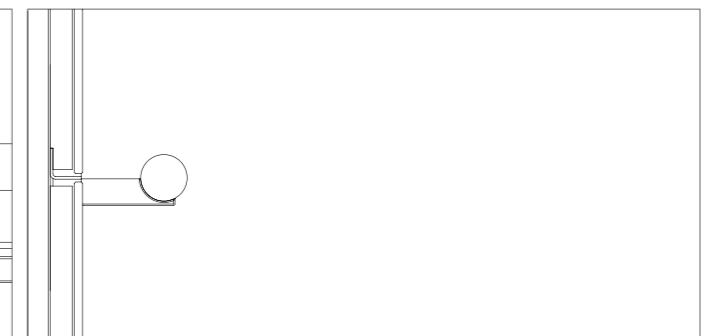
Corte vertical do painel lateral, lado do corrimão Apoio do corrimão.
